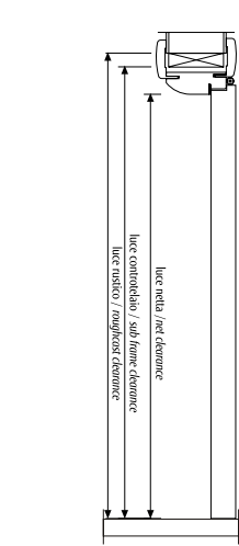
Sezione verticale / Vertical Section
