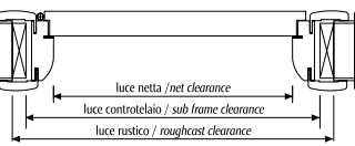
Sezione orizzontale / Horizontal section
