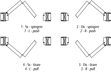
Sensi di apertura pieghevole / Folding door opening
