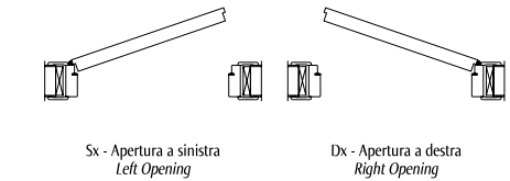
Sensi di apertura scorrevole a parete / Sliding to wall opening
